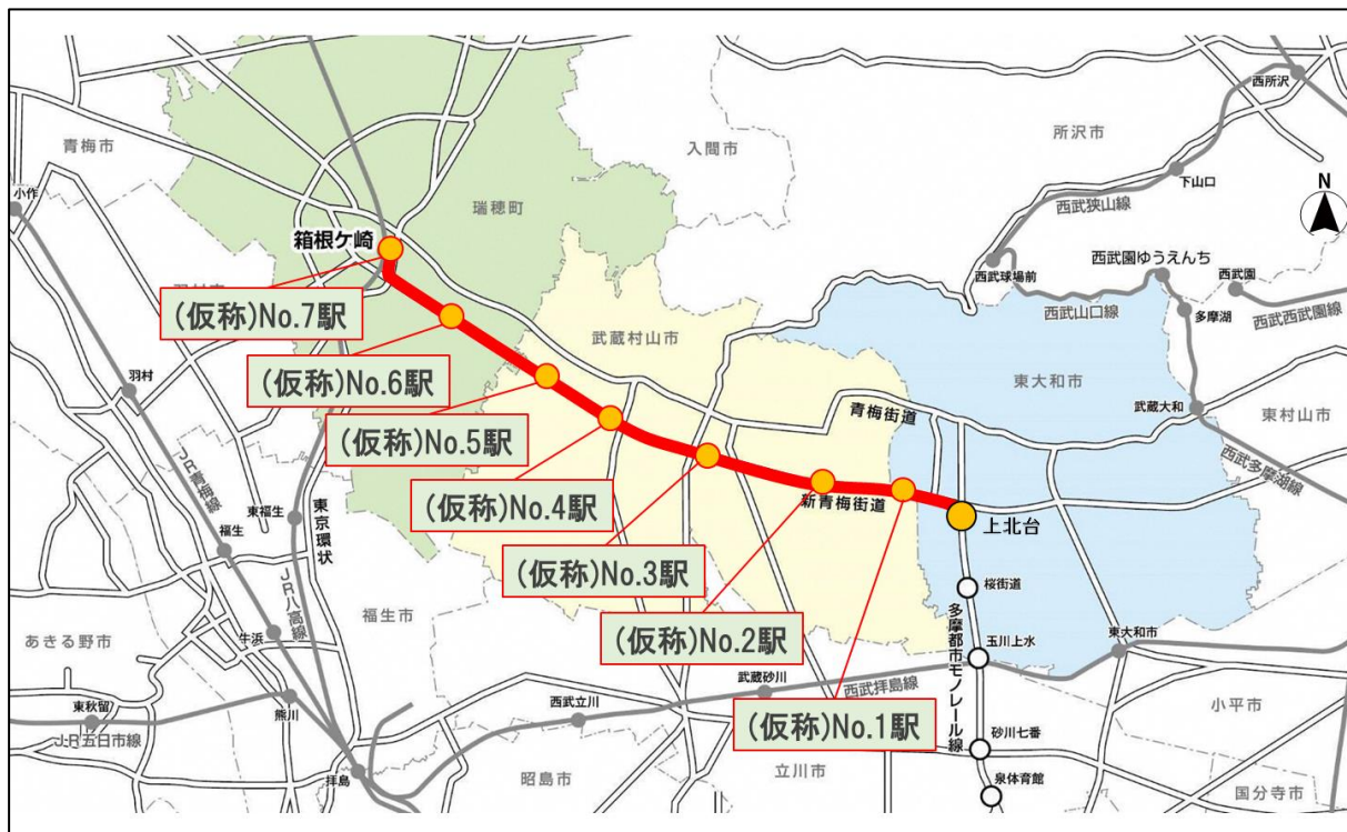
多摩都市モノレール延伸区間と新駅位置図
